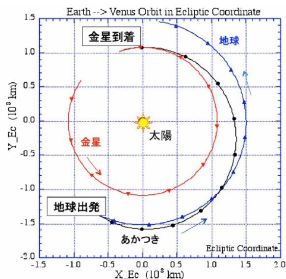
上: ロケットから分離される「あかつき」 下: 「あかつき」の金星到着は12月頃
