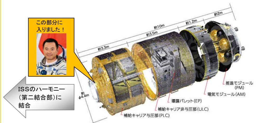
宇宙ステーション補給機「こうのとり」3号機の外観図
